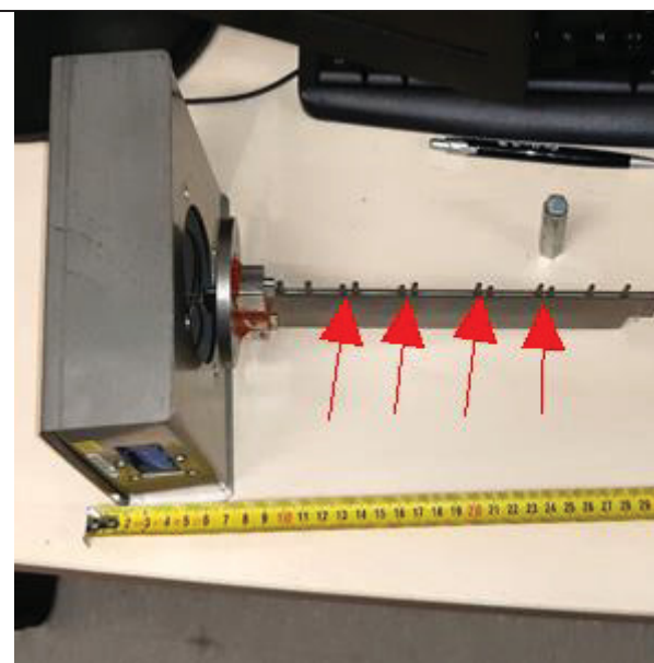
celková délka cca 300 mm, délka měřicí části cca 200 mm; termočlánky označené šipkou
