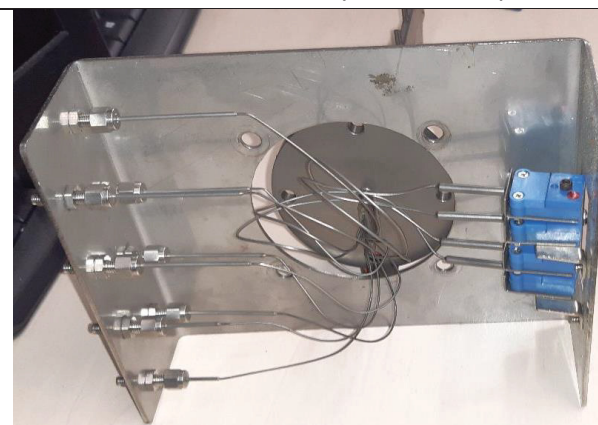
pohled na termočláňkové minikonektory zevnitř
