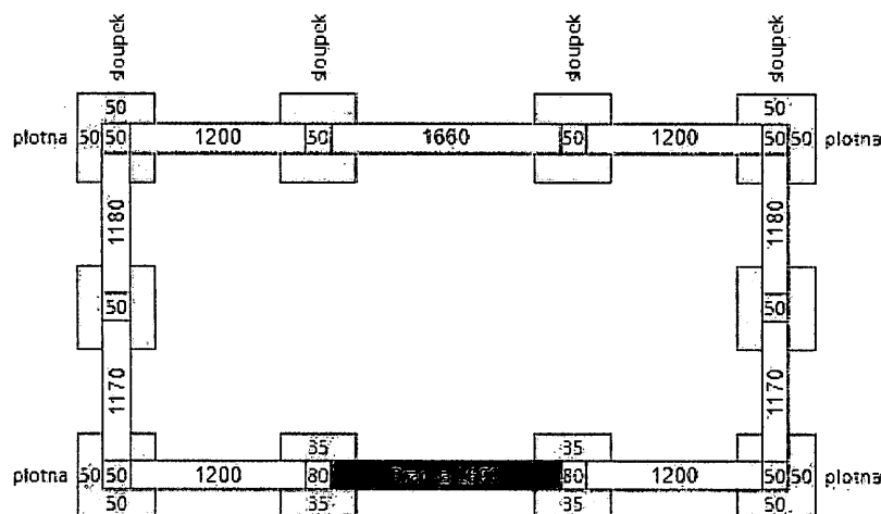
1) Kontejnerové stání kotvené do země - 4360x2600x1600 mm včetně branky
