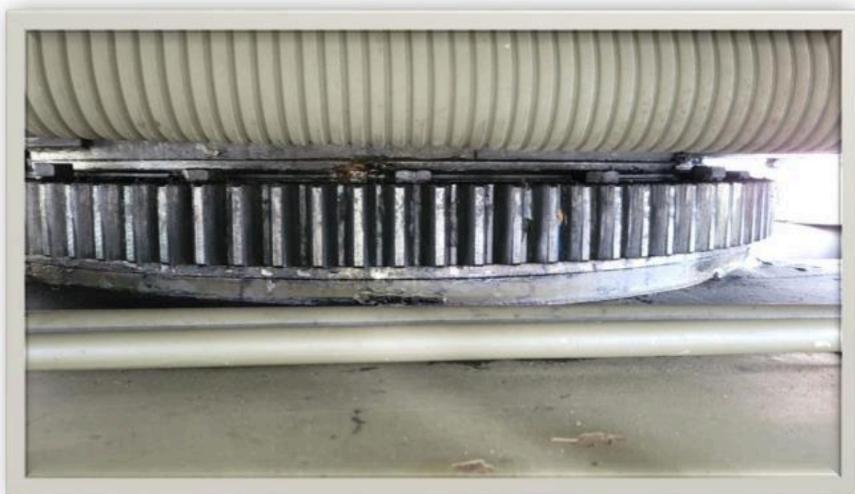
P-2 Prává strana - 2. svar
