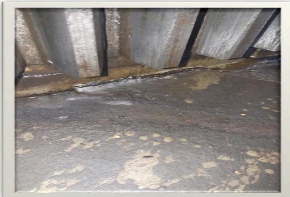
L-4 Levá strana - 4. svar – nahoře
