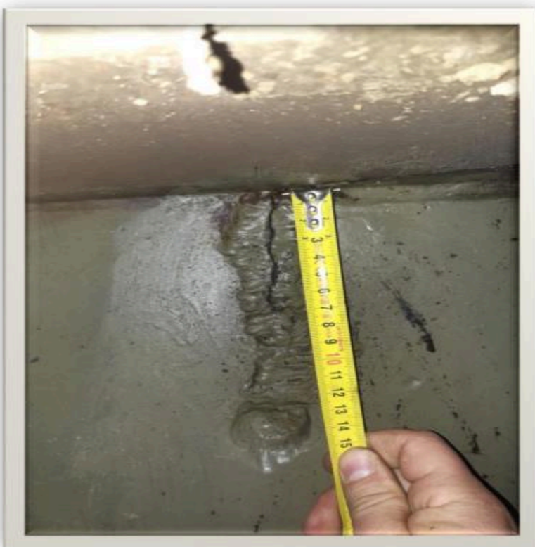
L-7 Levá strana - 7. svar – rám – detail
