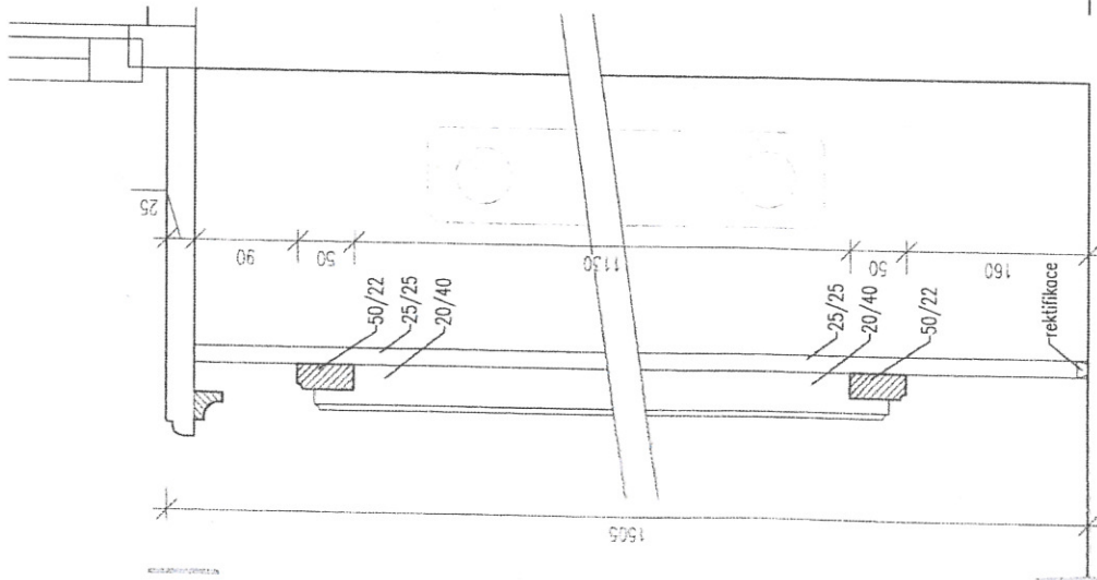
ŘEZ B (1:5)
