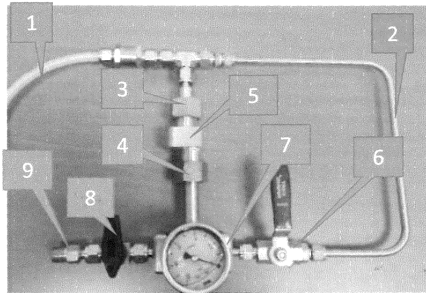
Obr. 5. Aplikační sestava (1-vstup dusíku, 2-by-pass, 3-připojení plynné fáze, 4-připojení kapalně fáze, 5-spojka kapalně a plynně fáze, 6-ventil by-passu, 7-kontrolní manometr, 8-hlavní uzavírací ventil, 9-výstup produktu)
