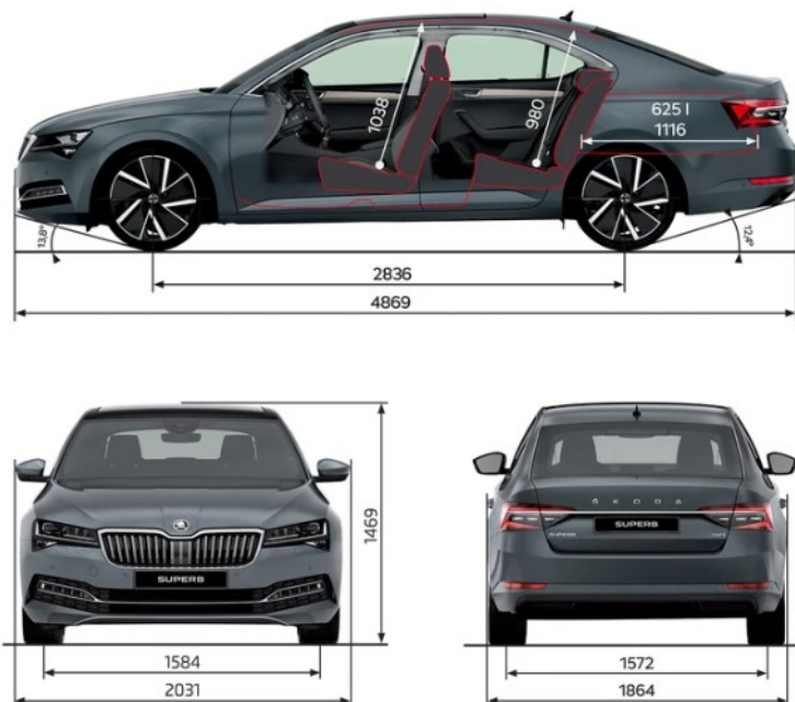
Rozměry nabízeného vozu
