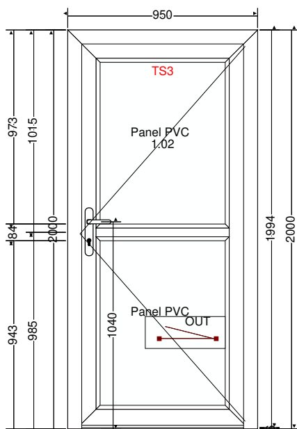
Vnitřní pohled
