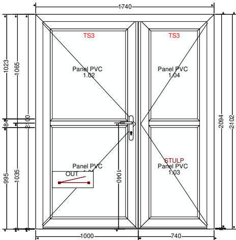
Vnitřní pohled
