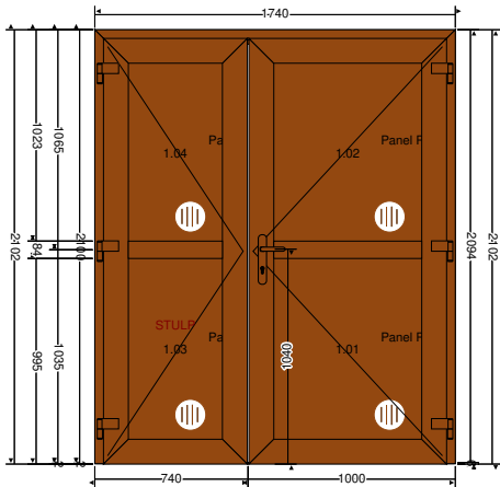
Vnitřní pohled
