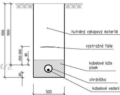
Vzorový schem. příčný řez kabelovou trasou dle ČSN EN 33 2000-5-52 ed.2
