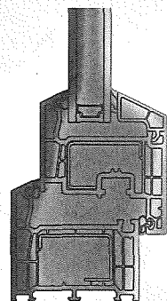
Průběh izoterm
