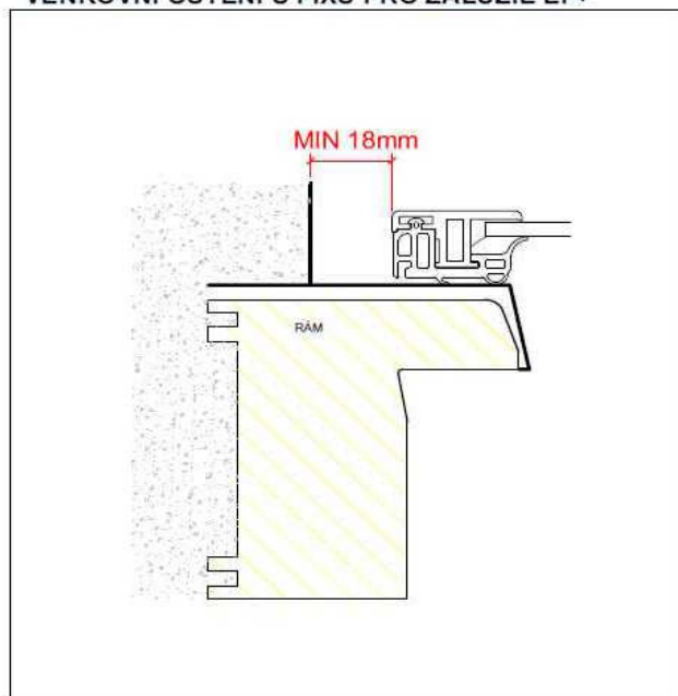
VENKOVNÍ OSTĚNÍ U FIXŮ PRO ŽALUZIE EF+
