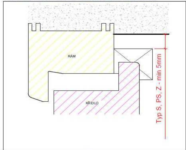
LOŽE A OSAZENÍ VNĚJŠÍHO PARAPETU
