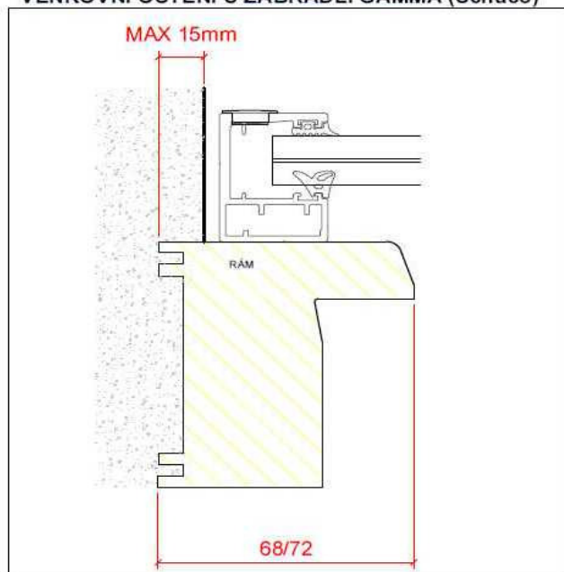
VENKOVNÍ OSTĚNÍ U ZÁBRADLÍ GAMMA (Schüco)
