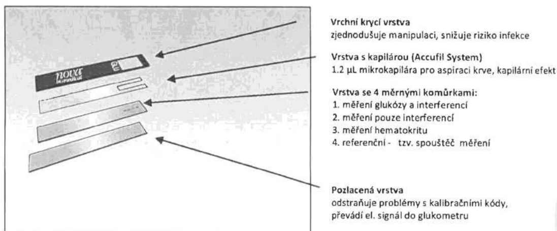
Obr. 1: Technologie MultiWell™ - unikátní koncepce testovacího stripu: 4 vrstvy, 4 měrné komůrky
