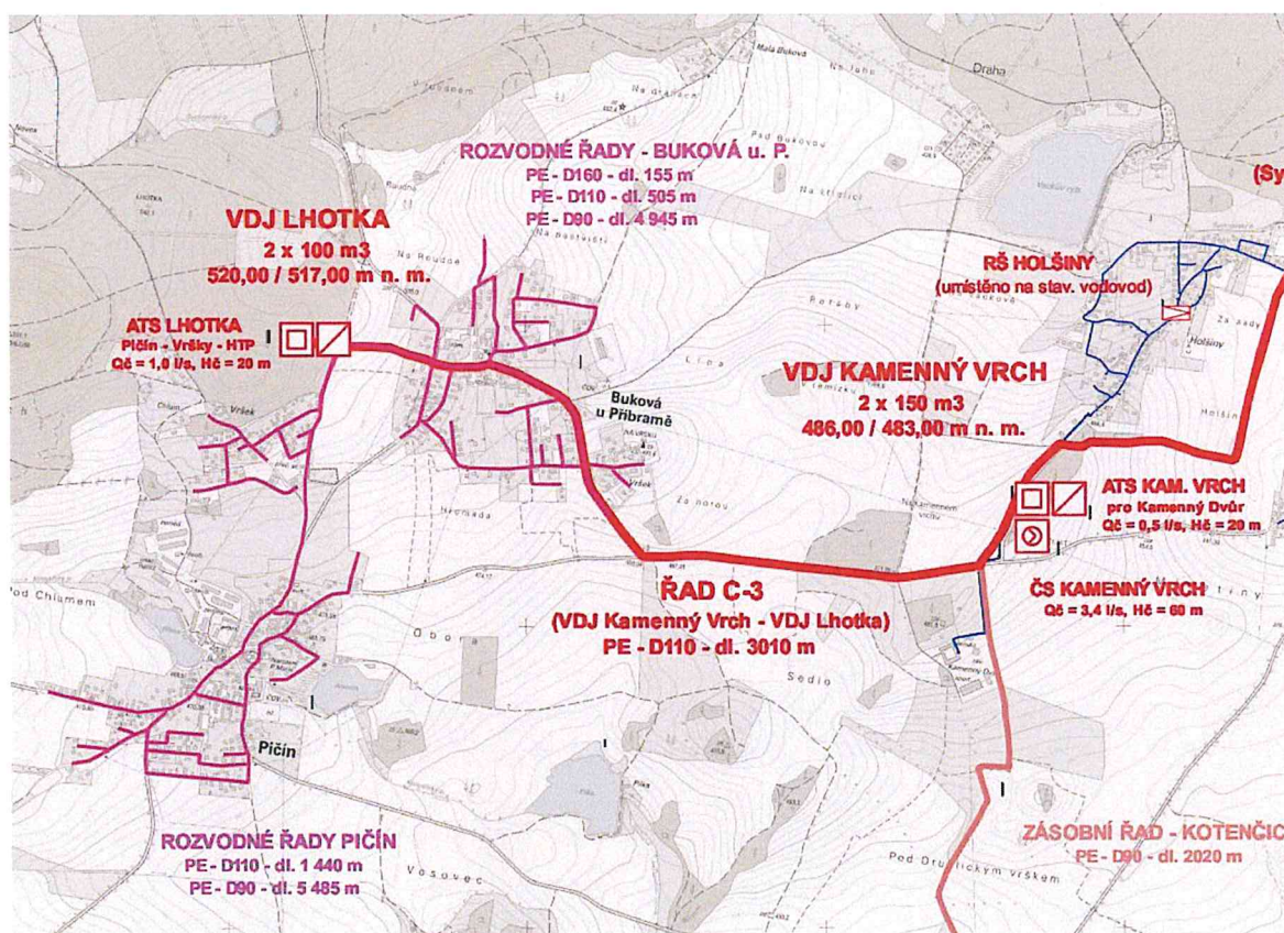
Obr. 1 Uvažované řešení zásobení obcí Buková u. P. a Pičín dle studie z roku 2021
