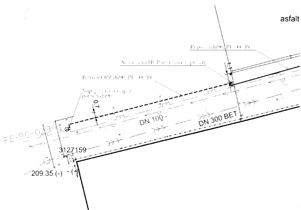
Půdorys (výřez ze situace) včetně zakreslení umístění objektu HUP
