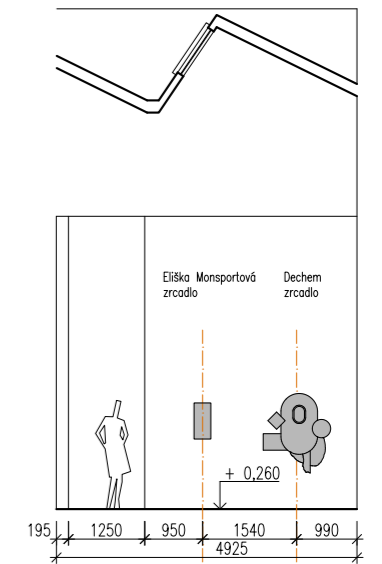
Pohled E
