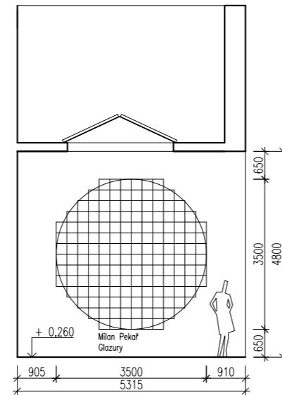
Pohled D
