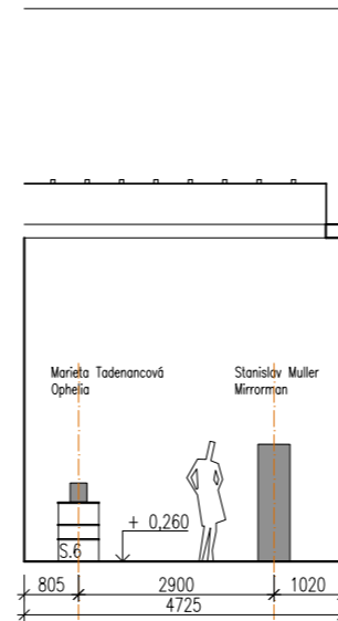
Pohled G
