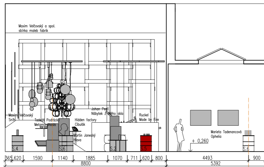
Řez CC'
