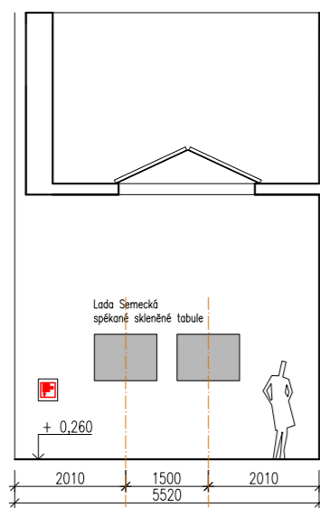
Pohled B
