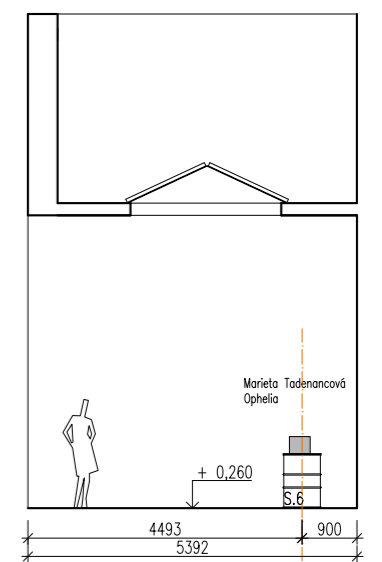
Pohled J
