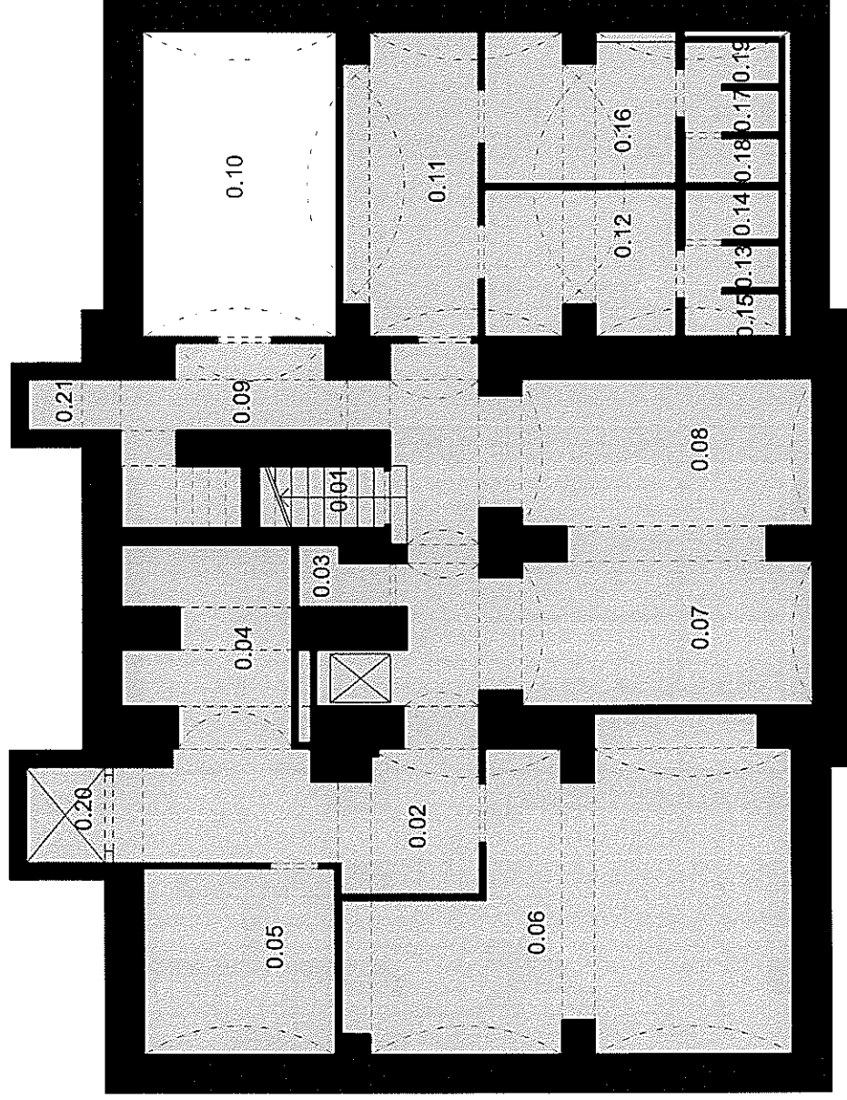
Schematický půdorys 1.PP
