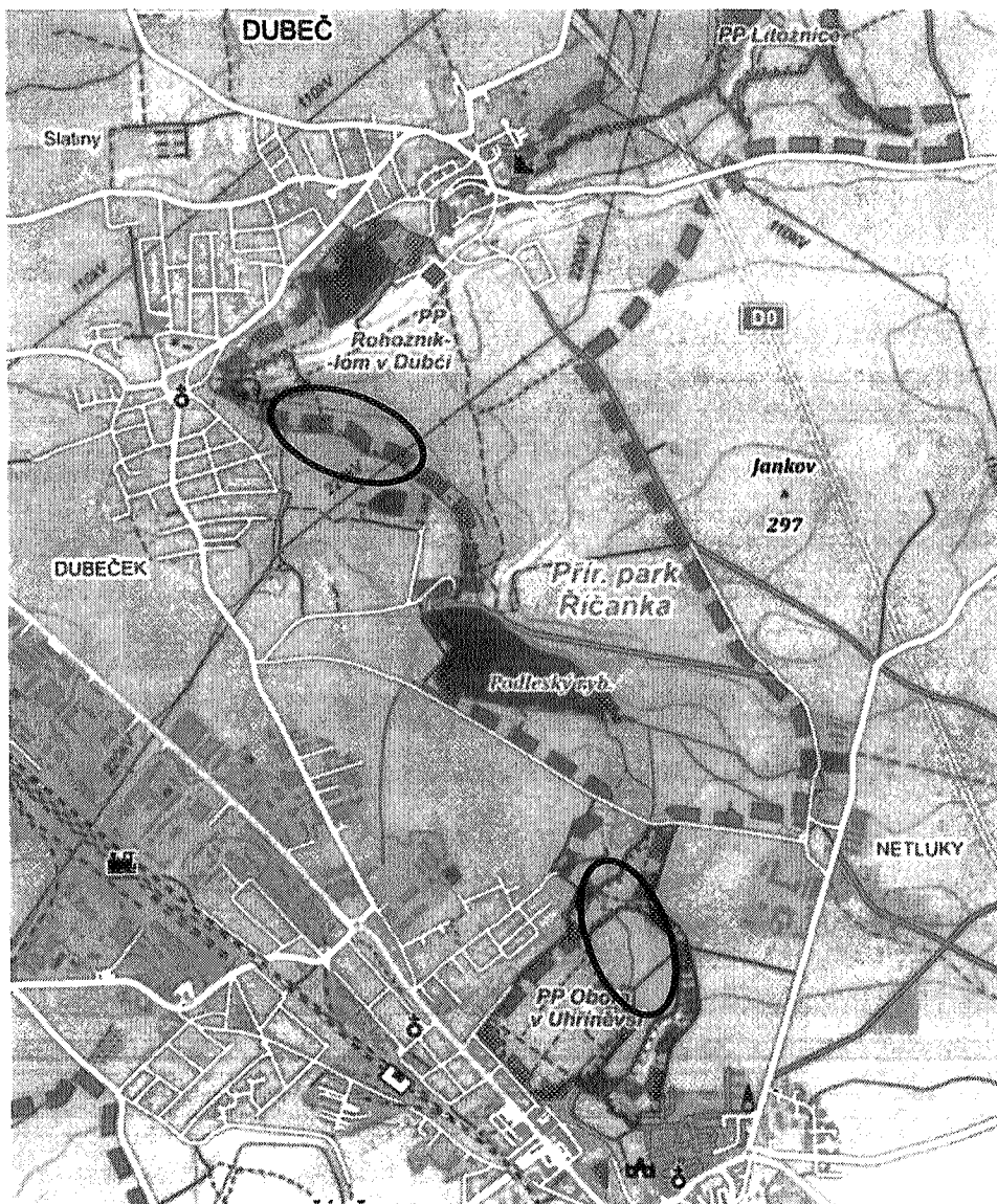
Obrázek 1 - místo předpokládaných profilů retenčních nádrží na Říčanském potoce
