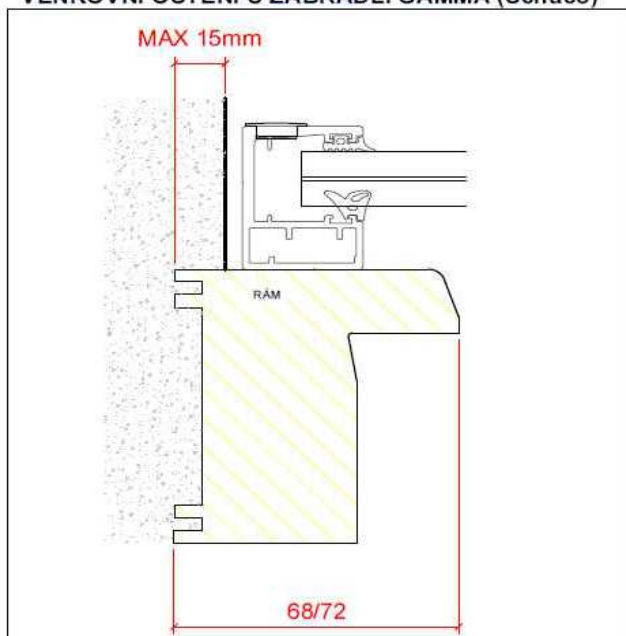
VENKOVNÍ OSTĚNÍ U ZÁBRADLÍ GAMMA (Schüco)
