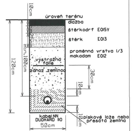
řez výkopem chodník, kabel NN/VN
