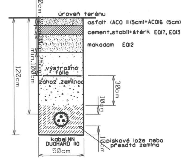
řez výkopem v asfaltové komunikaci kabel VN
