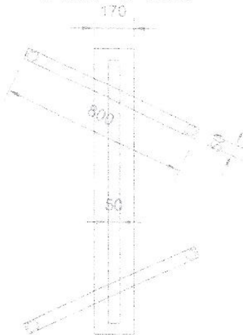
POHLED SPODNÍ
