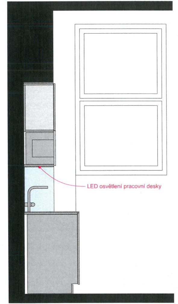
řez F
