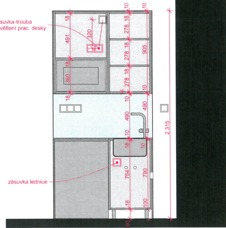
řez E
