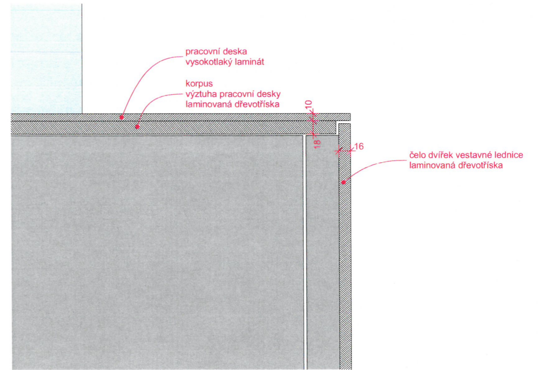
detail D3
