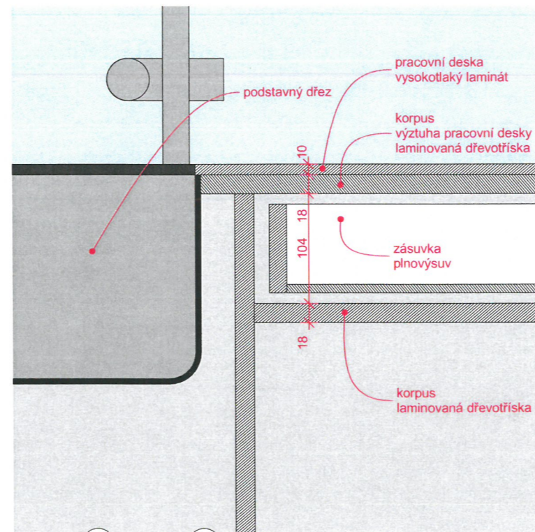
detail D2
