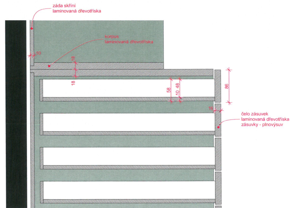
detail D5
