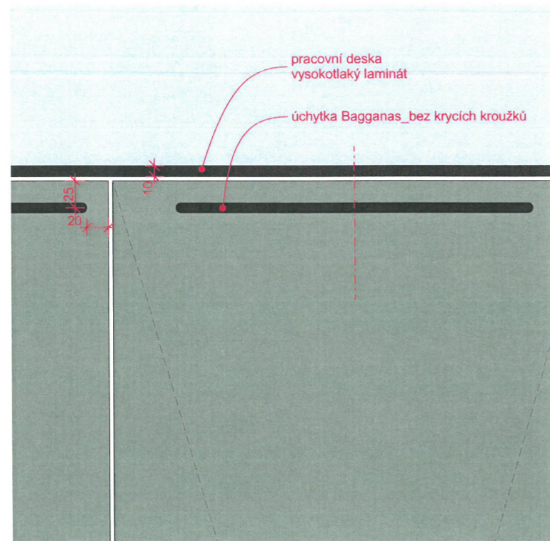
detail D1
