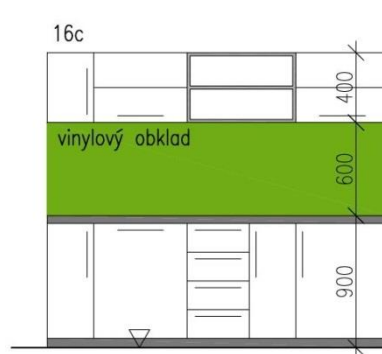
ČELNÍ POHLED
