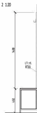
ŘEZ 2 1:20
