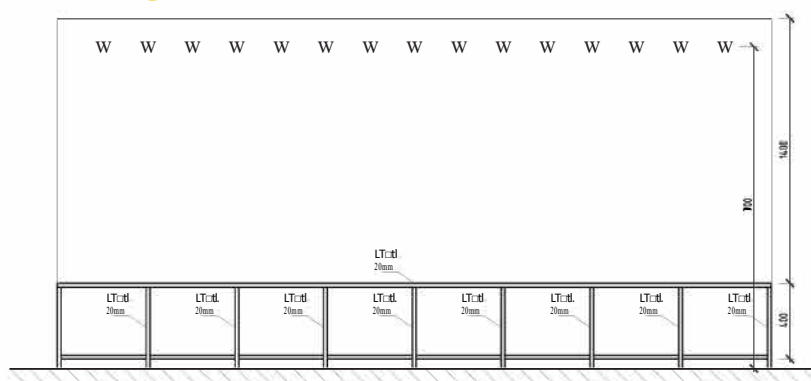
ČELNÍ POHLED 1:20
