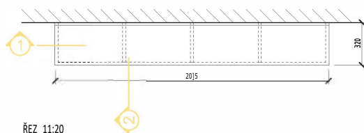
ŘEZ 11:20
