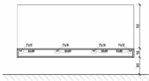
ŘEZ 11:20
