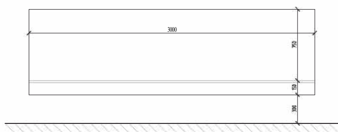
ČELNÍ POHLED 1:20
