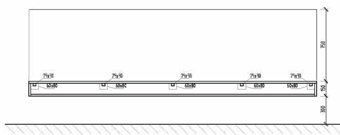
ŘEZ 11:20
