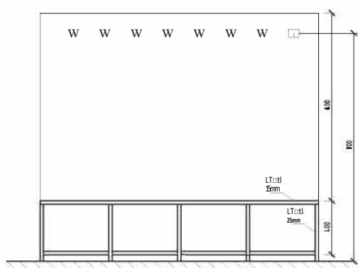
ČELNÍ POHLED 1:20
