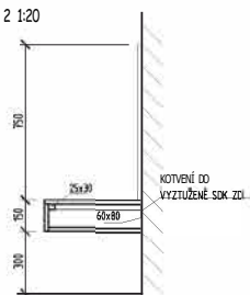
BOČNÍ POHLED 1:20
