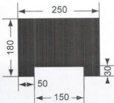
Obrněný transportér (terč č. 13)
