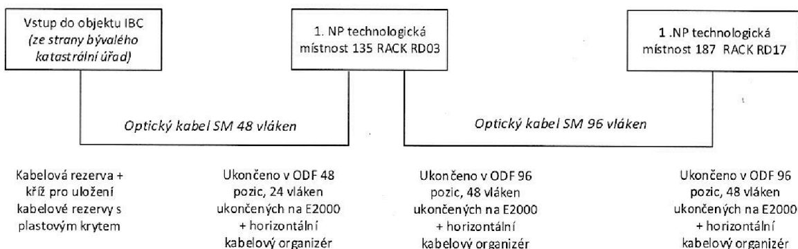
obr. Schéma s požadavky na trasy
