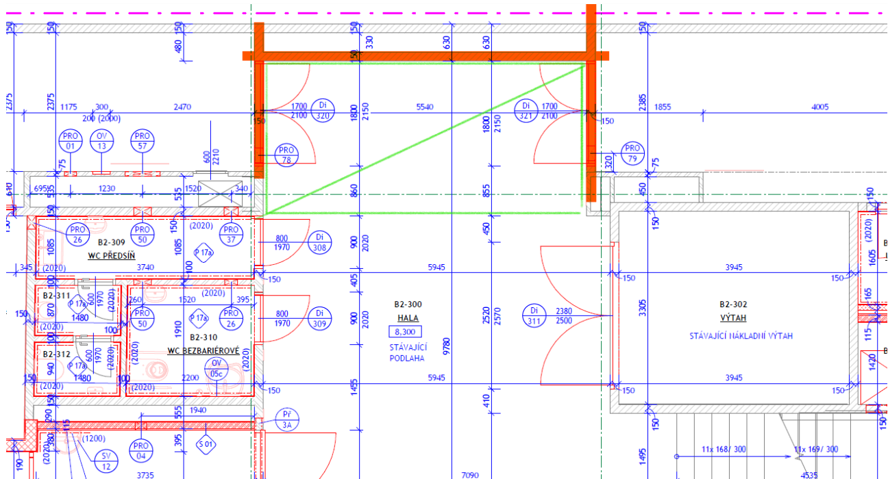
Schéma zadržek a nového SDK protipožárního podhledu pro typické podlaží
