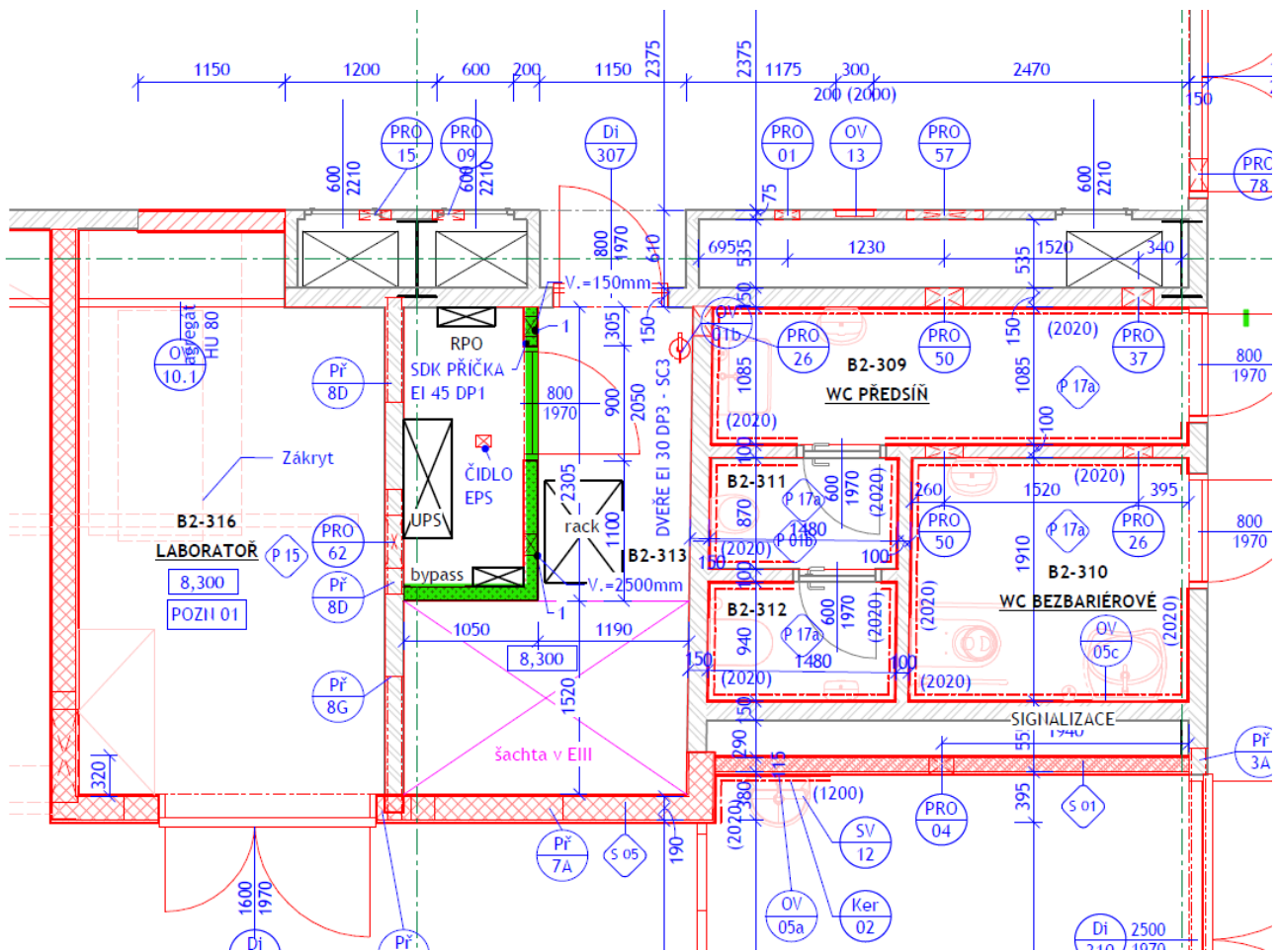
Schéma 3.NP
