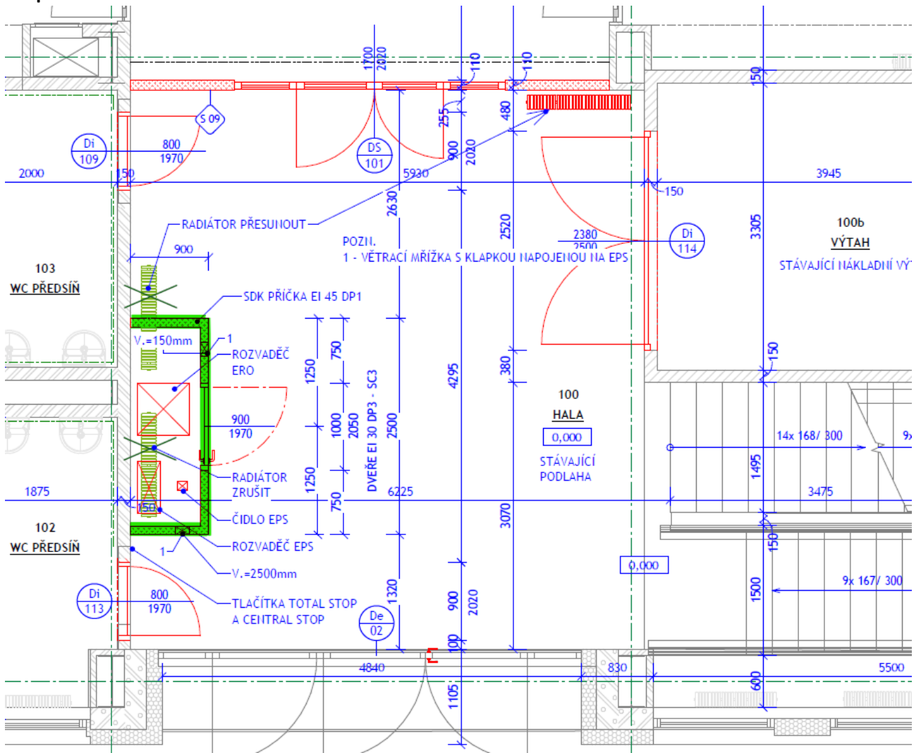
Schéma 1.NP
