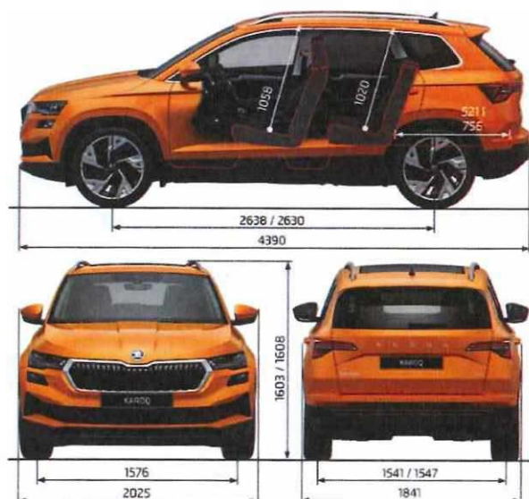
Rozměry nabízeného vozu
