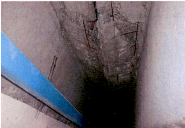
pohled nosné konstrukce nájezdové rampy v oblasti spodního MZ
