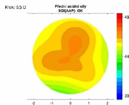
Centrální strmá rohovka na centrální topografii* (pacient s předchozí hypermetropickým LASIK/PRK)
