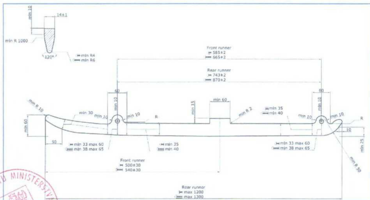
Obr. 2 – Technická specifikace
