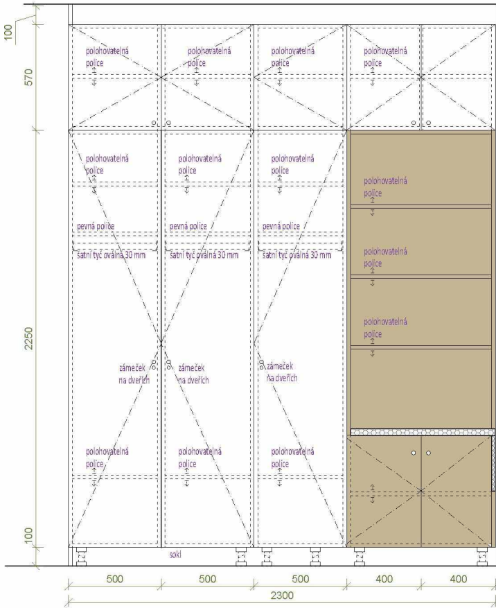
POHLED a
