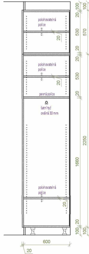
ŘEZ A-A
