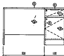
POHLED PŘEDNÍ M 1:20
