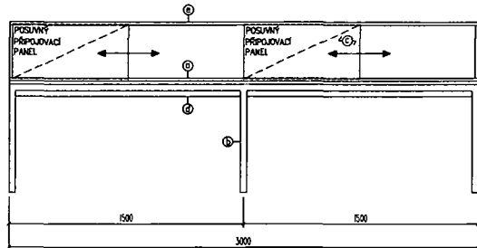
POHLED PŘEDNÍ M 1:20
