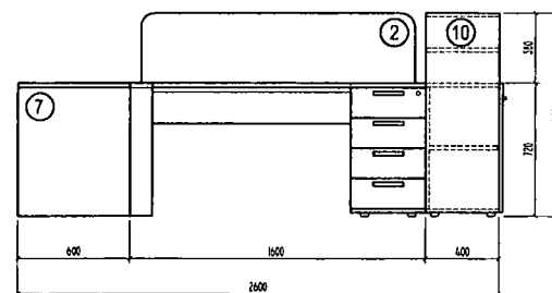
POHLED PŘEDNÍ
