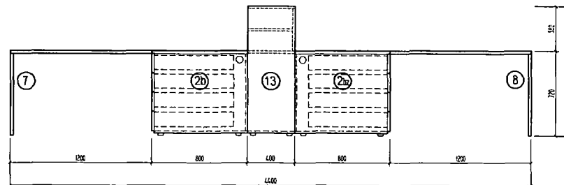
POHLED BOČNÍ
