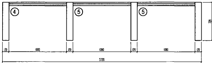
POHLED BOČNÍ
