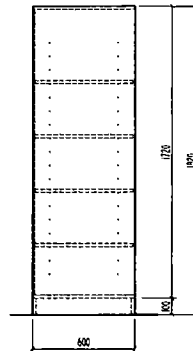
POHLED 2 M 1:30
