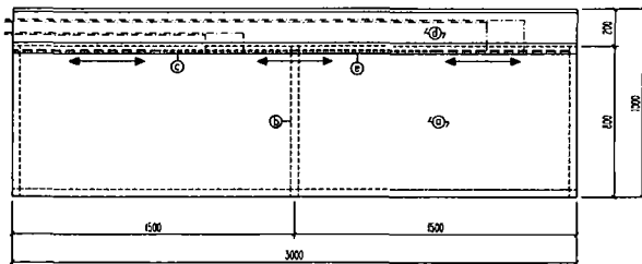
POHLED PŘEDNÍ M 1:20
