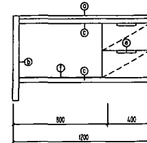
POHLED PŘEDNÍ M 1:20
