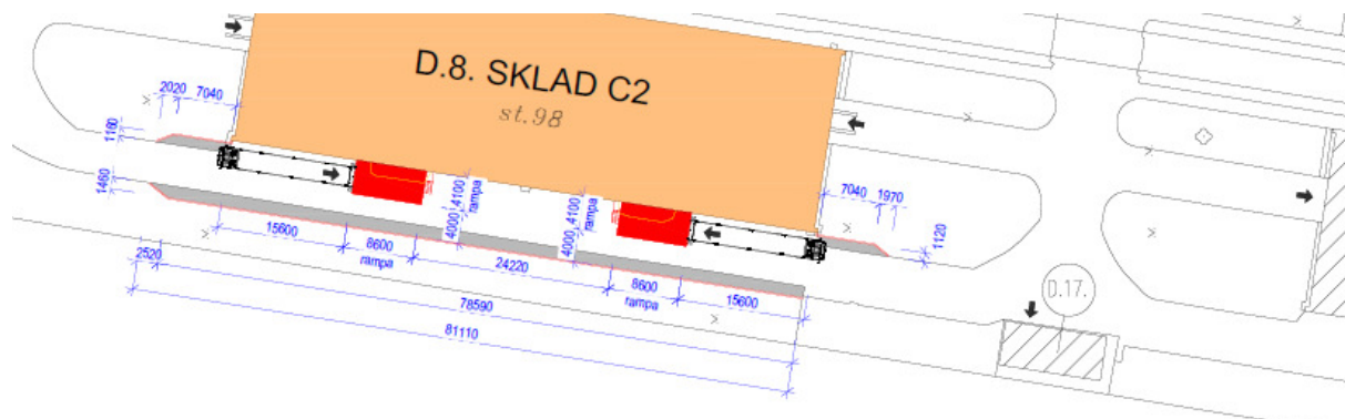
Obr. č. 2 – Schéma požadovaného rozšíření komunikace u skladu C2
