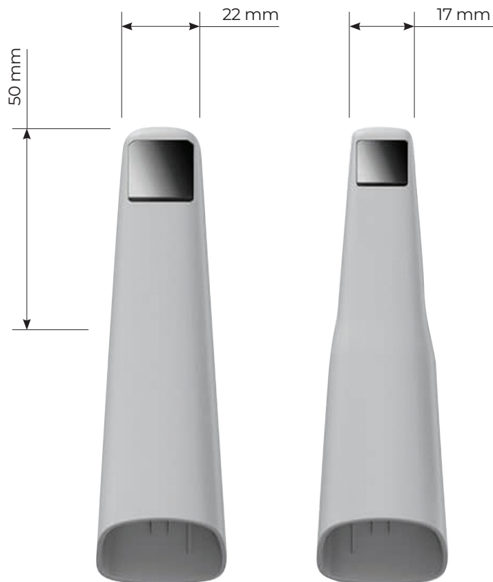
Standardní hlavice
