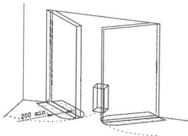
Obrázek C.5 – Dvoukřídlové kývavé dveře
