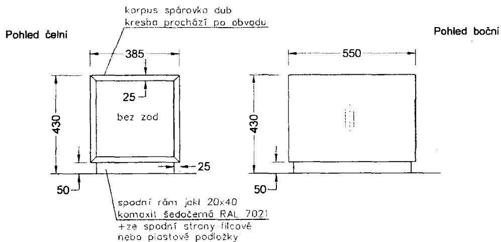
Půdorys
