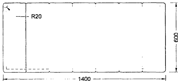
Půdorys
