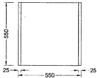
Půdorysný řez
