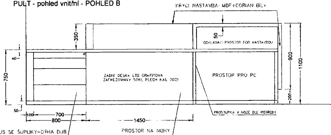
PULT - pohled vnitřní - POHLED B
