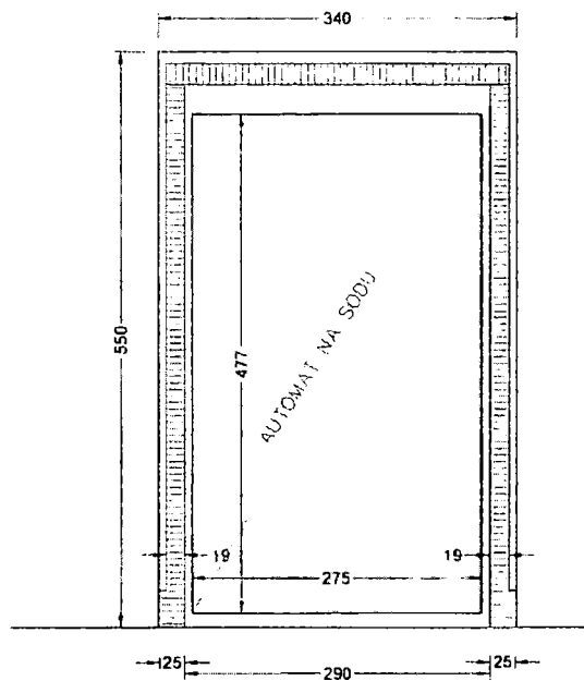
Půdorysný řez - m 1:5
