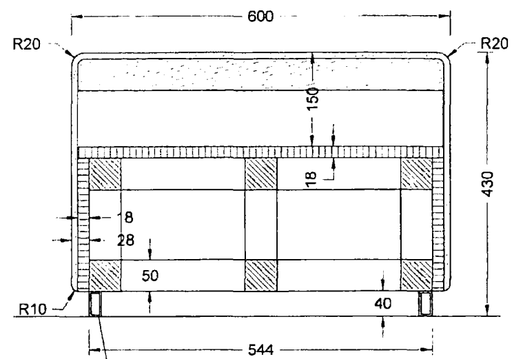
řez A - A
