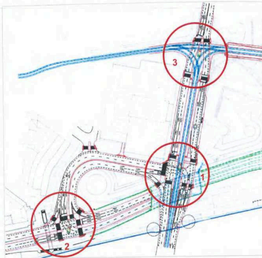
Obrázek 1. – Rozsah DIP
