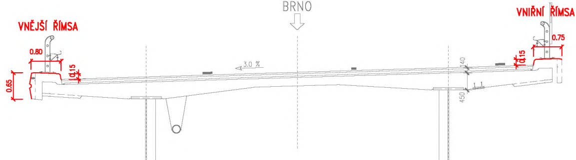
VZOROVÝ PŘÍČNÝ ŘEZ
