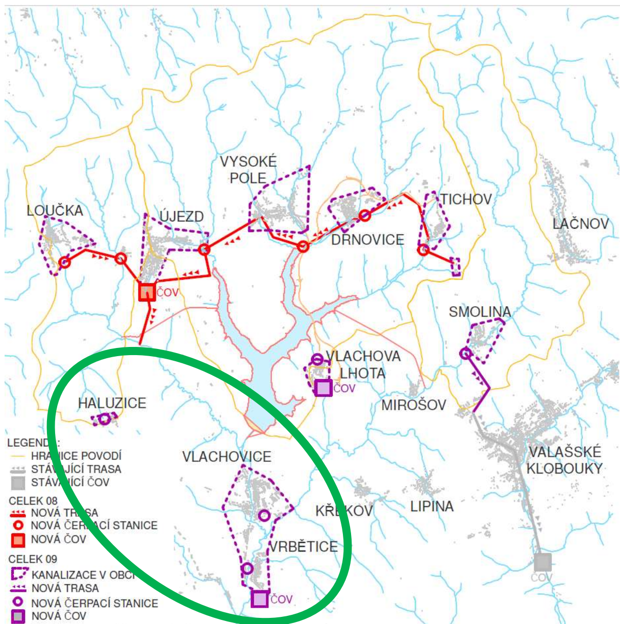
Obrázek 2: Schéma řešení nakládání s OV Celky 08 a Celky 09 zeleným oválem jsou vyznačeny obce v rozsahu tohoto technického zadání
