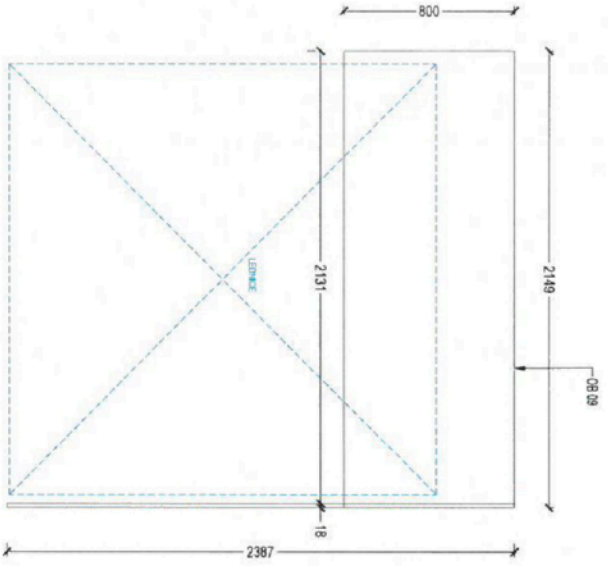
CELNÍ POHLED
