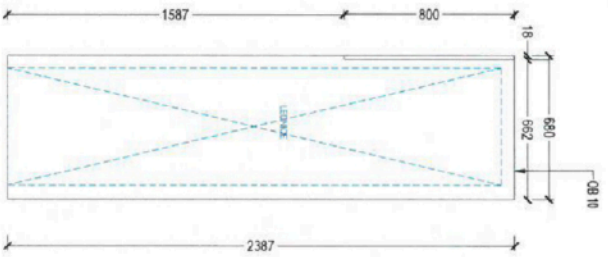
BOČNÍ POHLED
