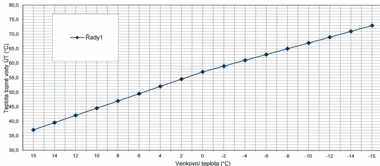
Teplotní křivka
