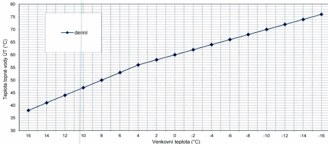
Teplotní křivka
