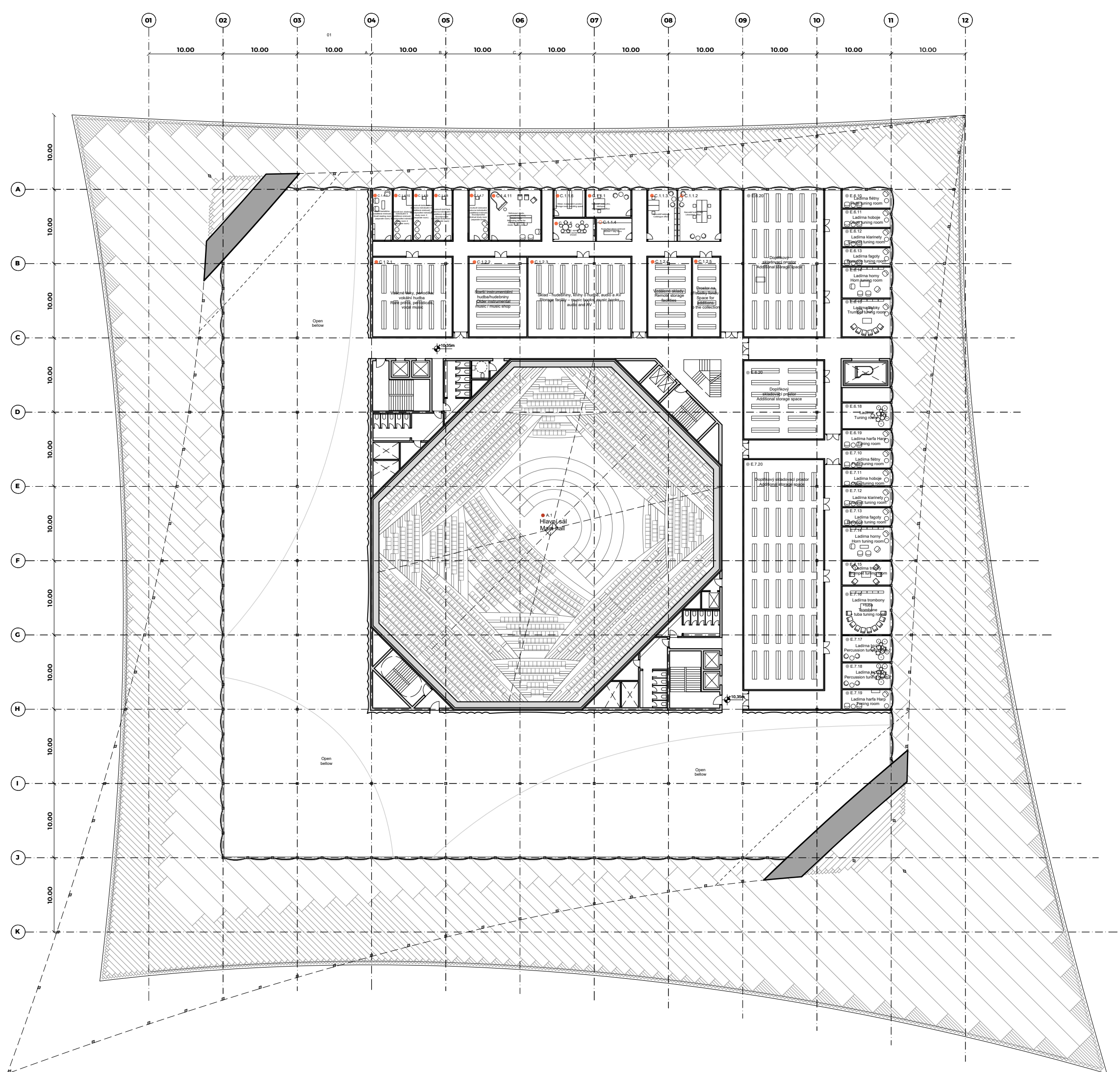
Level 4 Floor Plan Plán - 4. podzemní podlaží 1:500
