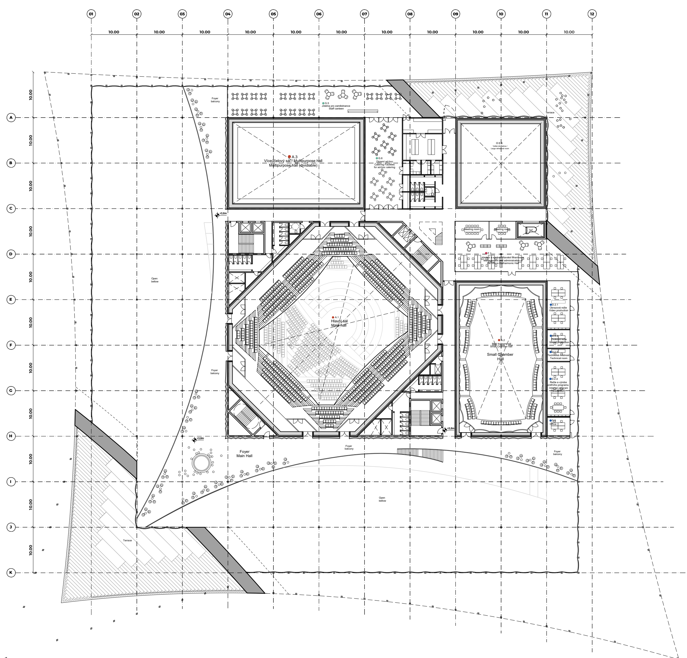
Underground Floor Plan Plán - 1. podzemní podlaží 1:500
