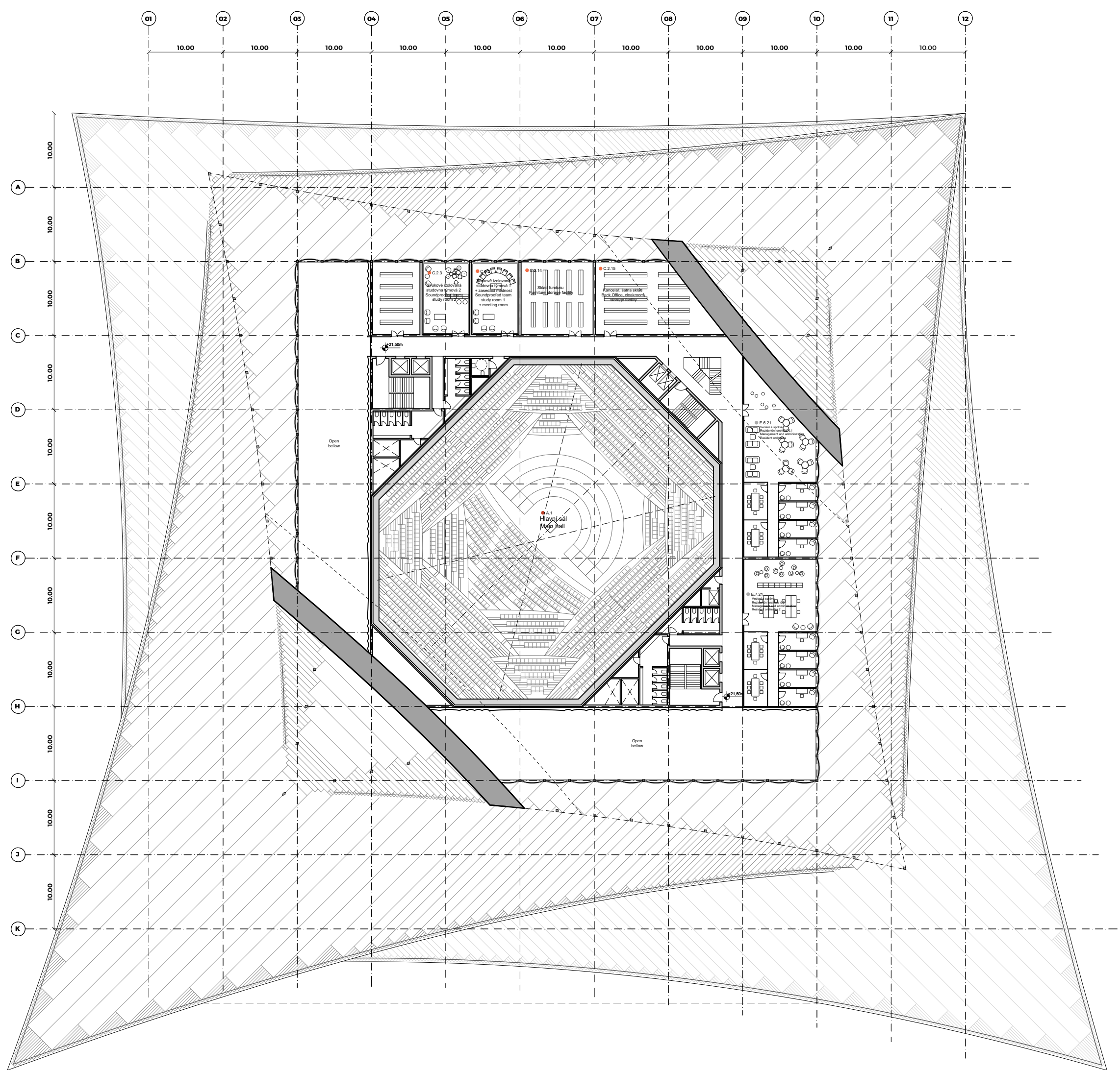
Level 6 Floor Plan Plán - 6. podzemní podlaží 1:500
