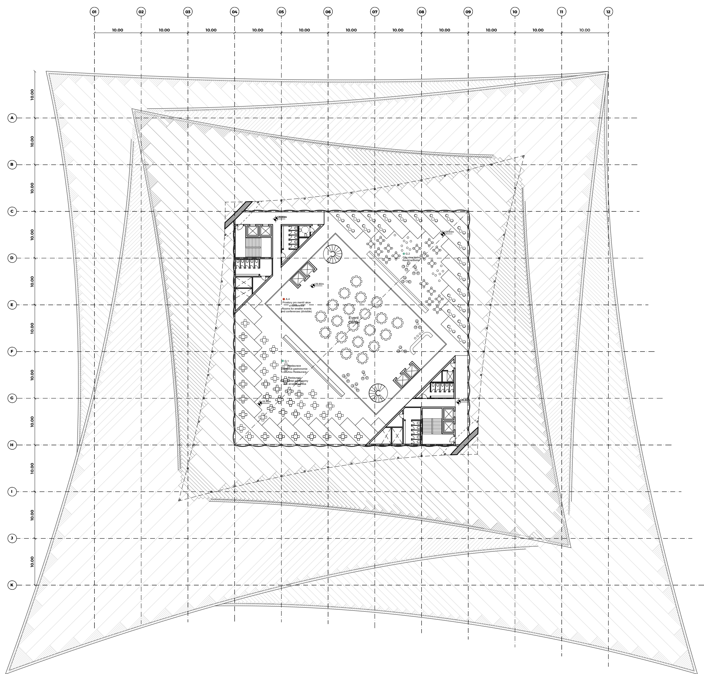
Level 7 Floor Plan Plán - 7. podzemní podlaží 1:500
