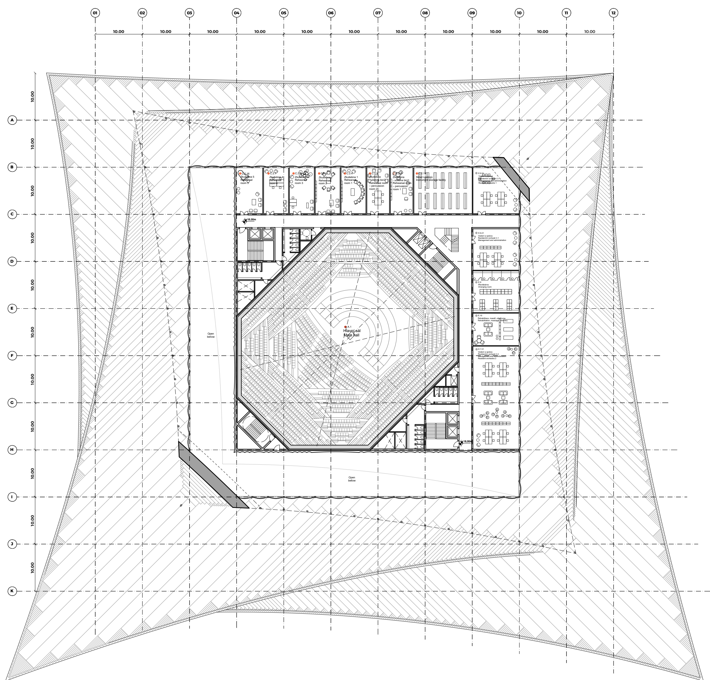
Level 5 Floor Plan Plán - 5. podzemní podlaží 1:500
