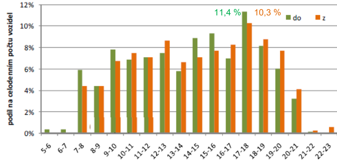
Obrázek 3 - Graf denní variace vjezdů a výjezdů VOZIDEL přes hranici lokality s vyznačením ŠH
