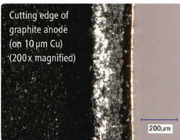
Obrázek 2 Zvětšený (200x) pohled na hrany materiálů připravené precizním nástrojem Cutting Pliers
