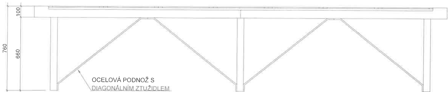
POHLED ČELNÍ
