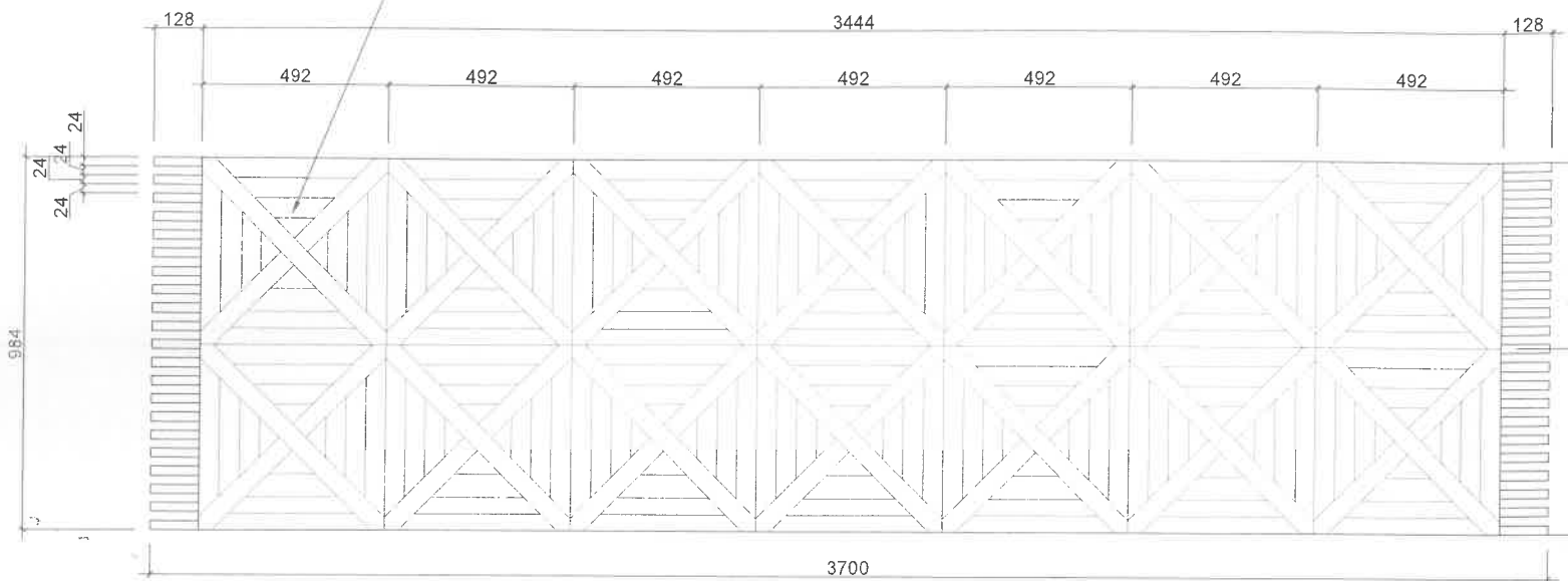
POHLED ČELNÍ
