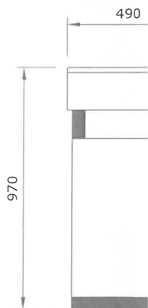
POHLED BOČNÍ
