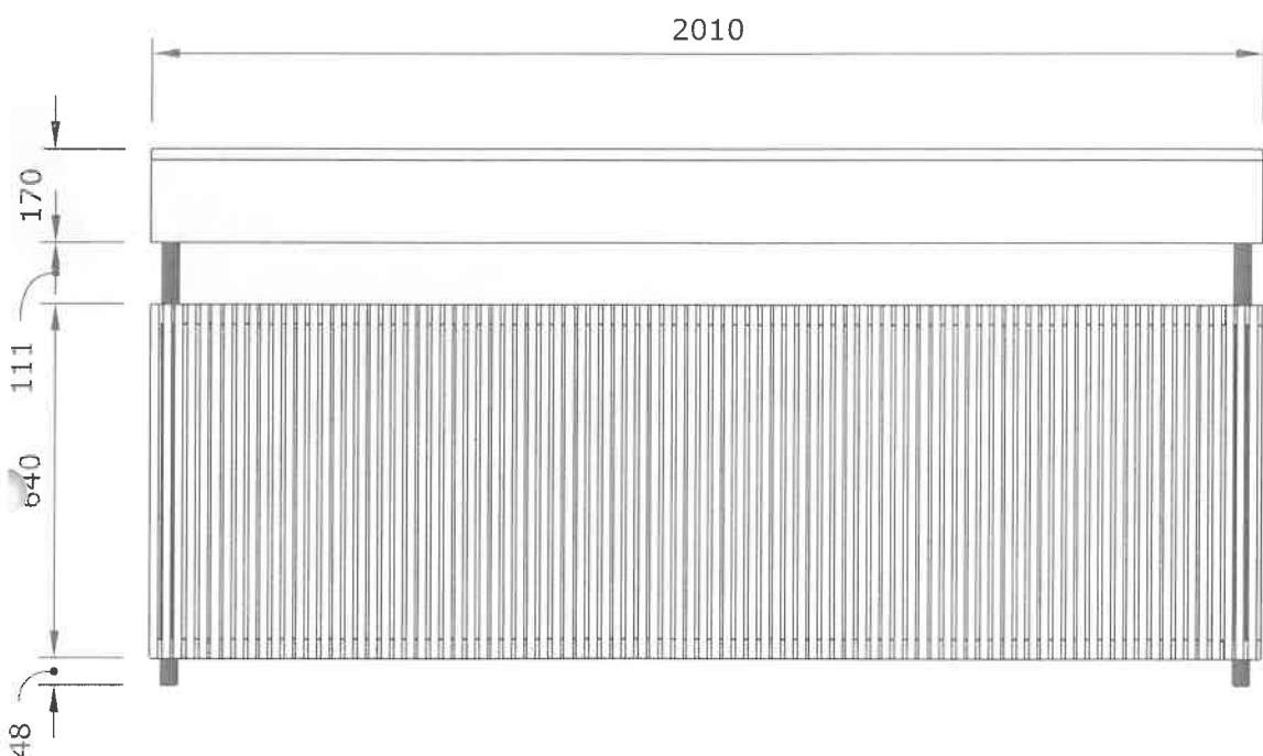
POHLED HORNÍ
