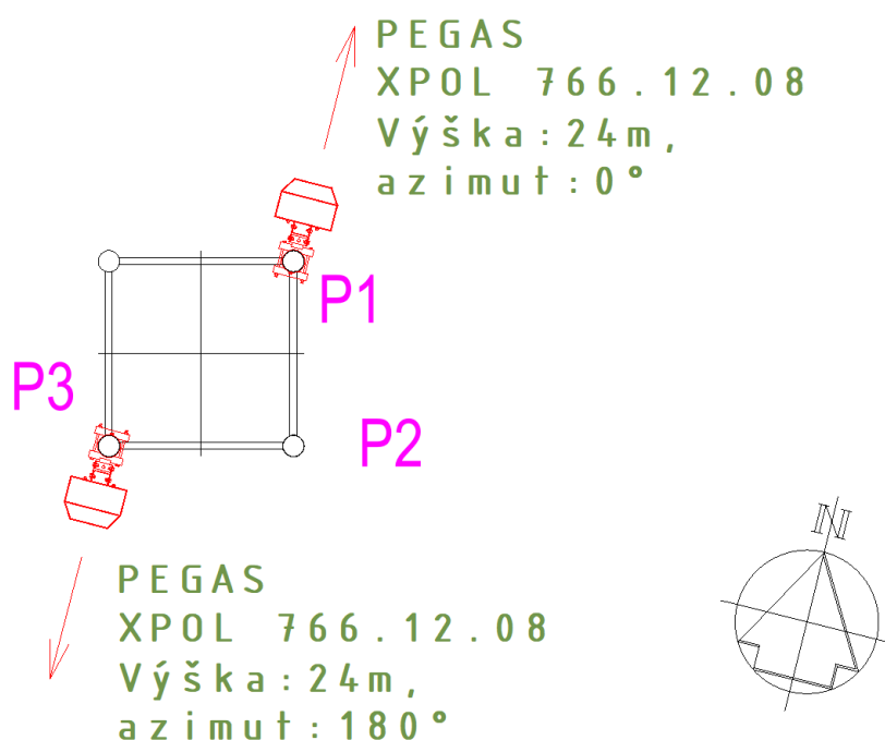
Obr. 6 Půdorys umístění antén
