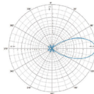
E-Plane | 425 MHz
