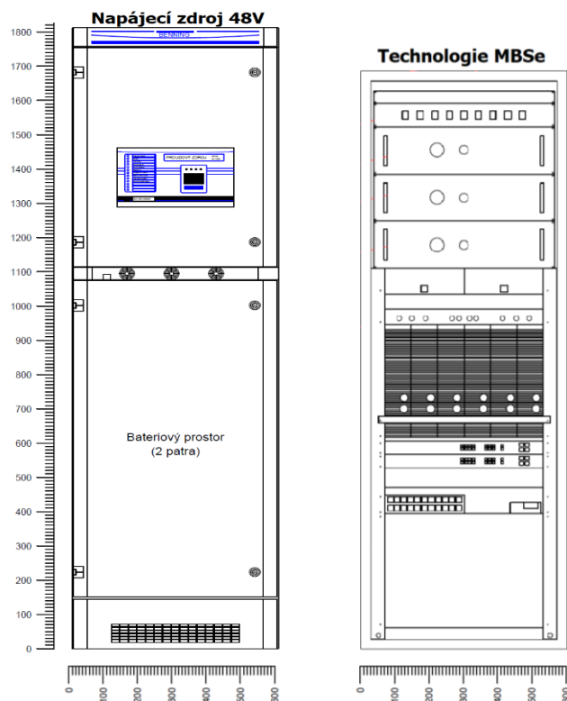
Obr. 2 – Rozměry technologických stojanů
