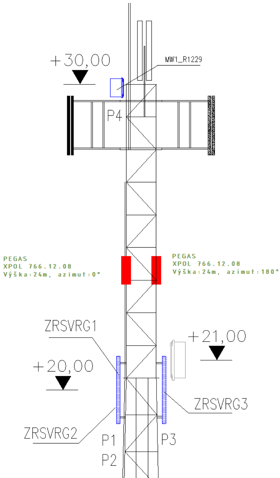
Obr. 6 Pohled na umístění antén
