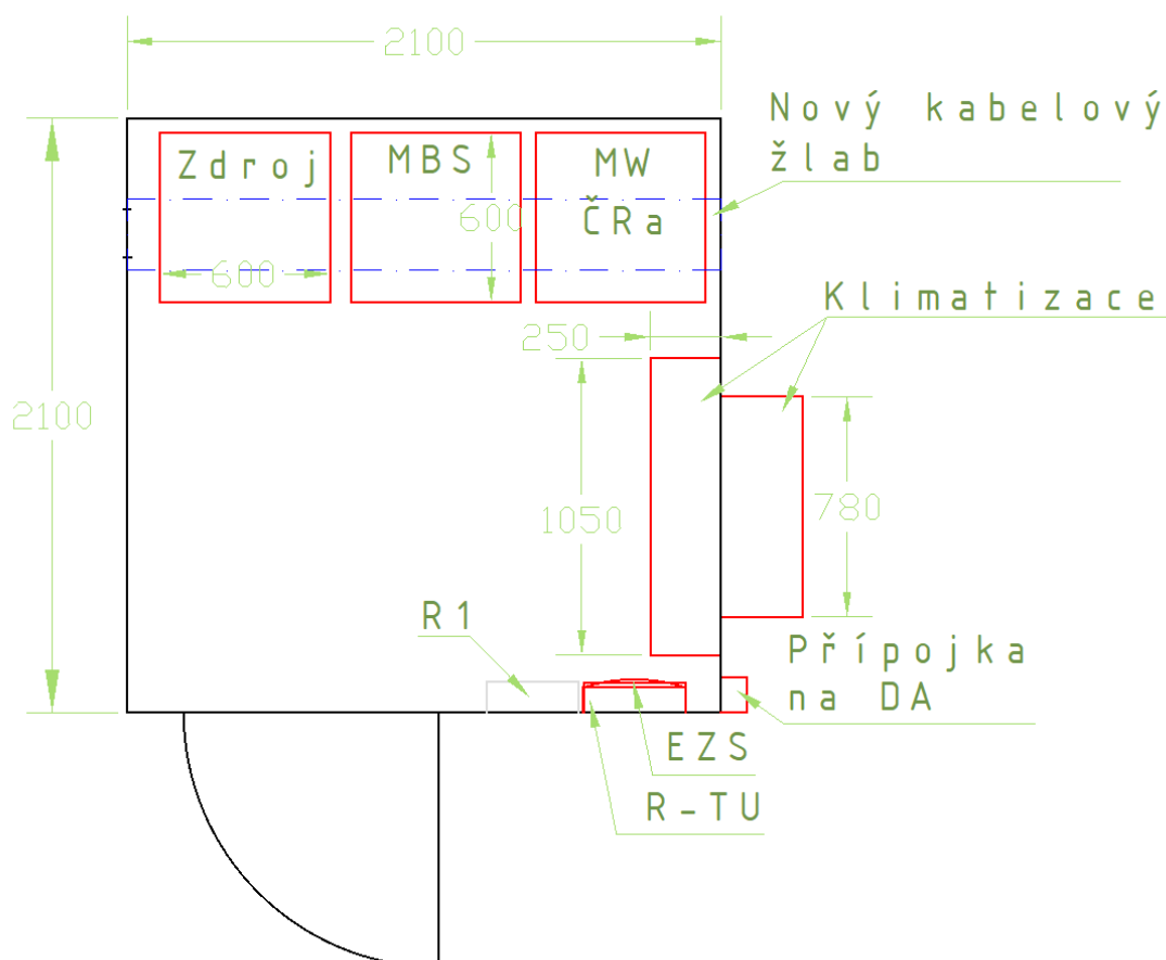
Obr. 3 Návrh umístění technologie
