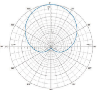
H-Plane | 425 MHz
