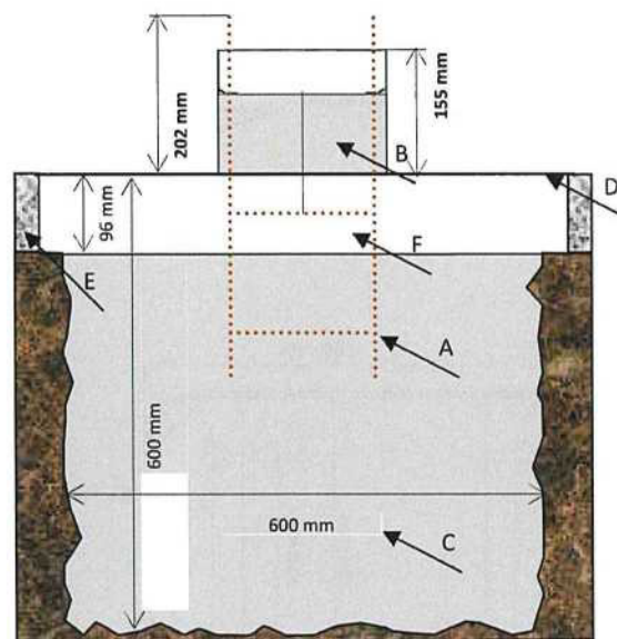
Varianta č. 4 (ovládací prvky ve výšce 1337 mm)
