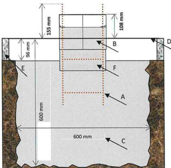
Varianta č. 3 (ovládací prvky ve výšce 1300 mm)
