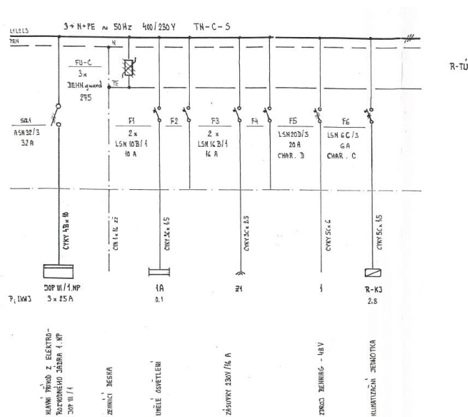
Obr. 4 – Příklad zapojení zdroje Benning
