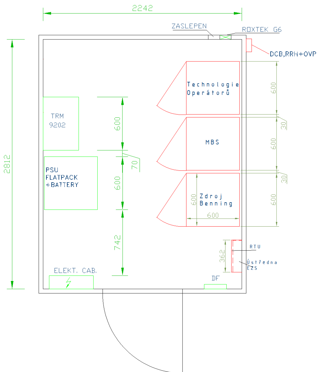
Obr. 2. - Půdorys rozmístění stojanů v kontejneru
