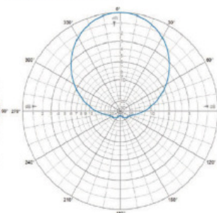
H-Plane | 425 MHz
