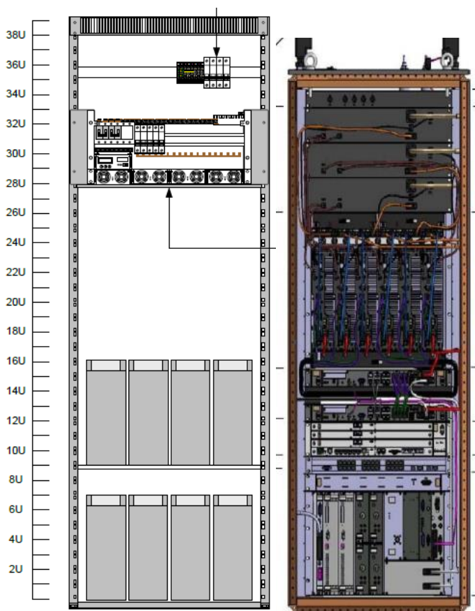
Obr. 3. – Technologické stojany
