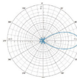
E-Plane | 425 MHz
