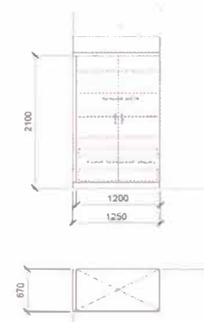
Místnost 128 - Plaz. 1
