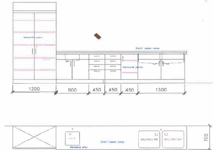
Místnost 127 - Poz 1
