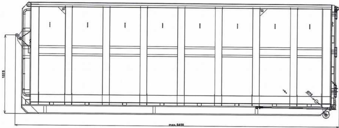
levá strana
