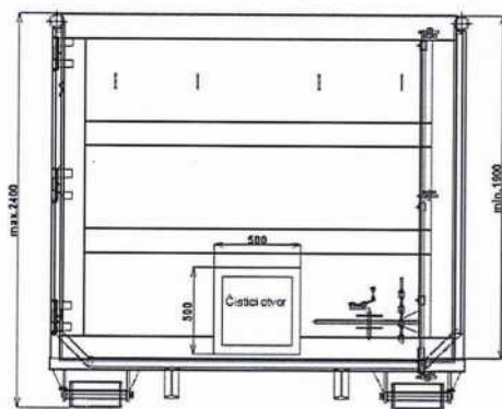
zadní pohled
