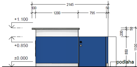
Pohled 4
