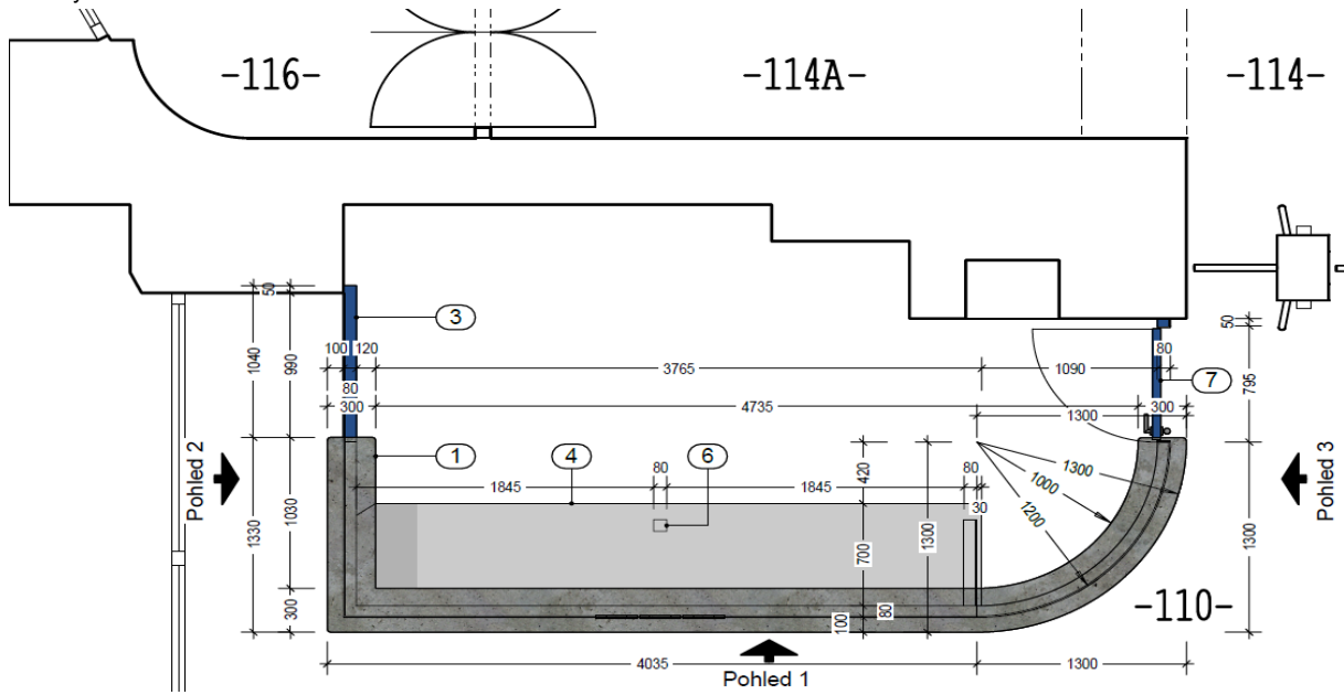
Půdorys
